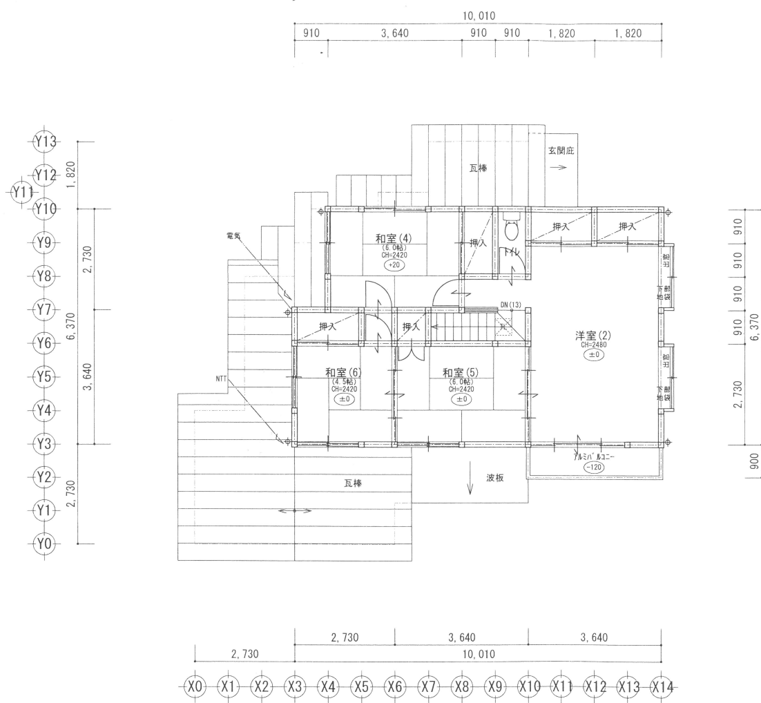
2階平面図
