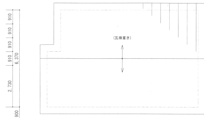
屋根伏図
