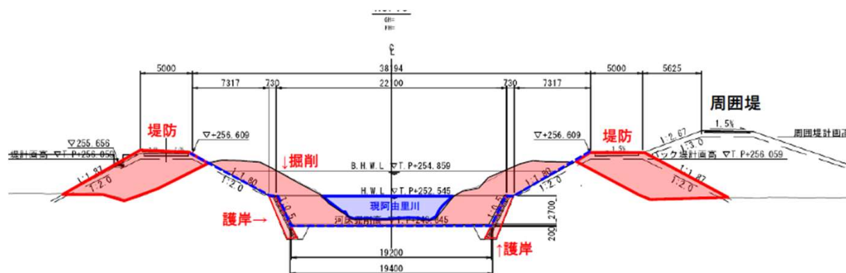
国工事区間の代表的な断面図
